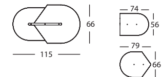
315.F.210A BEETLE CONFIG. 210A
