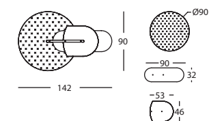
315.F.453E BEETLE CONFIG. 453E
