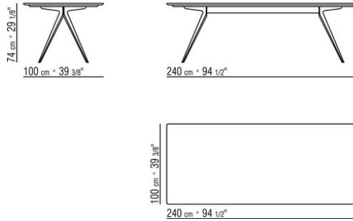
COD. 0238L6 TABLE
