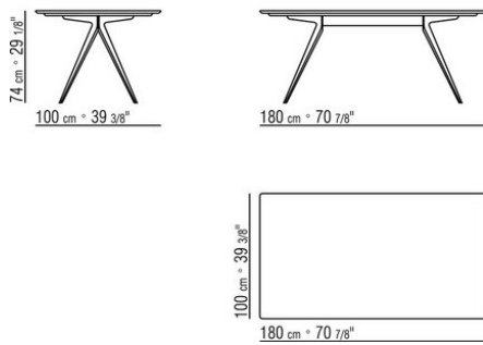
COD. 0238L7 TABLE
